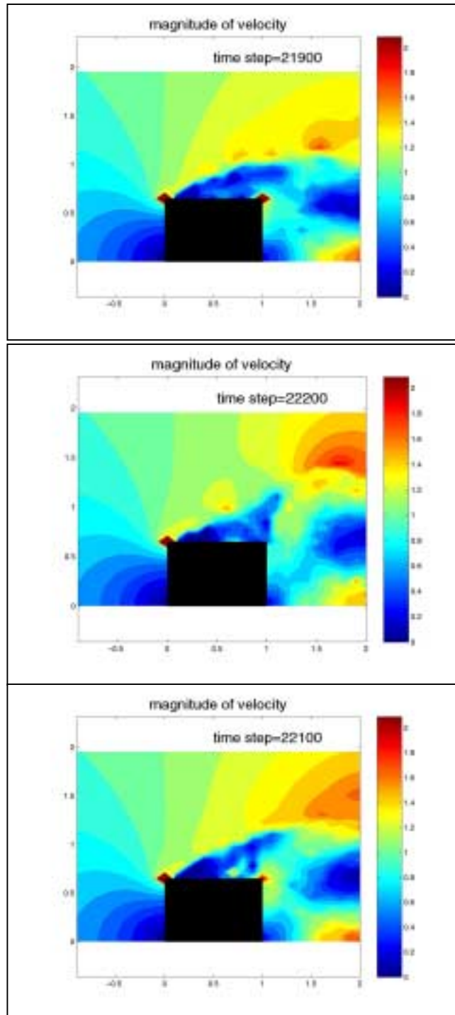
Fig. 4.8 Velocity magnitude
