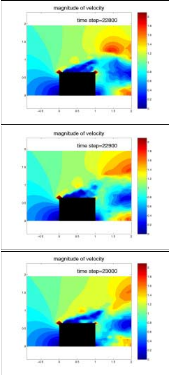
Fig. 4.11 Velocity magnitude
