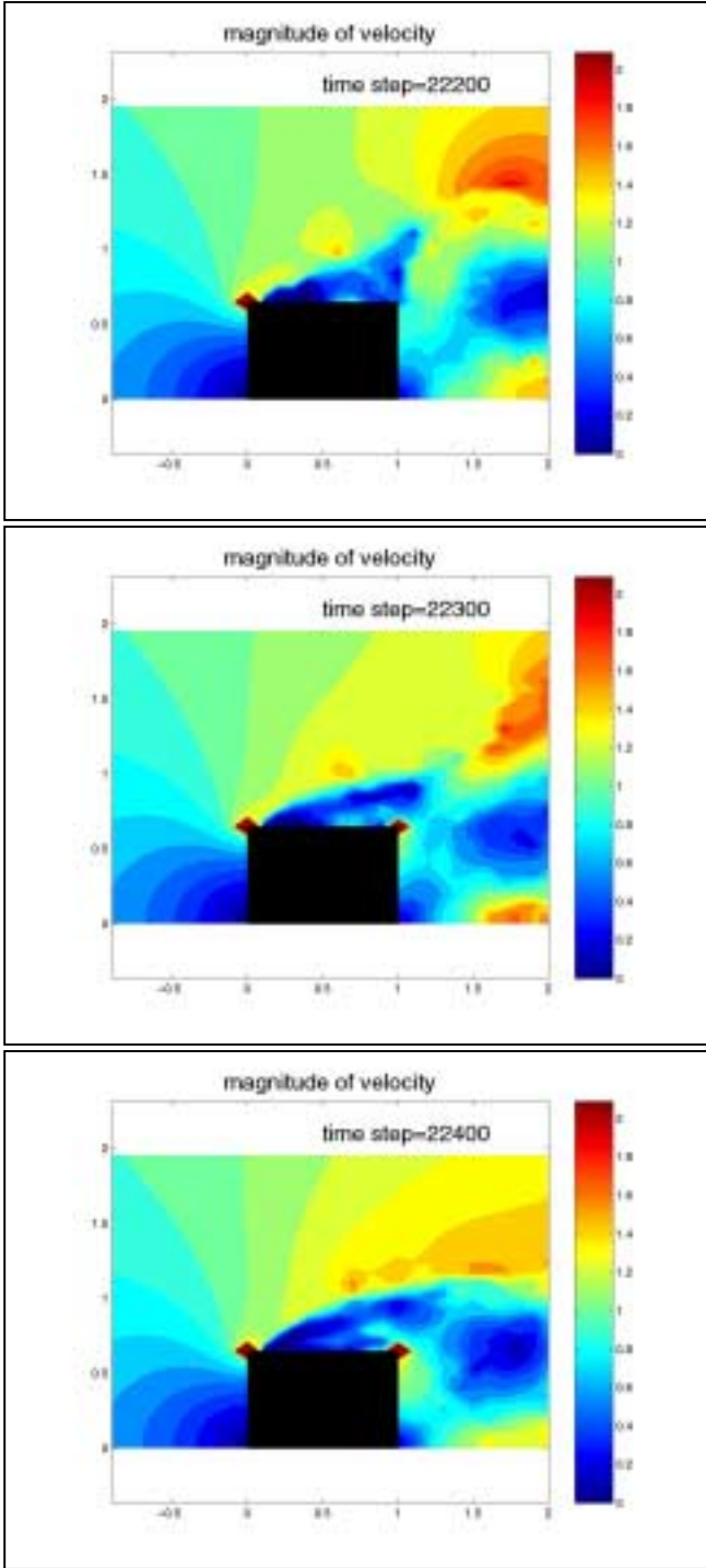
Fig. 4.9 Velocity magnitude
