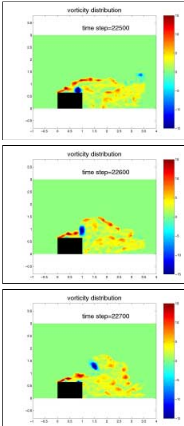
Fig. 4.17 Vorticity
