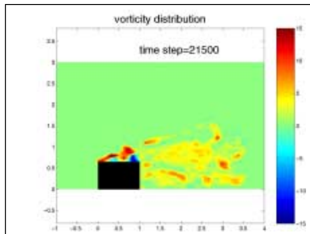
Fig. 4.13 Vorticity
