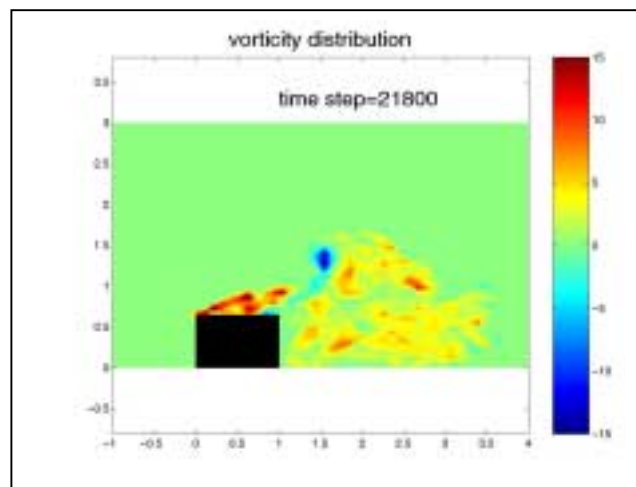
Fig. 4.14 Vorticity
