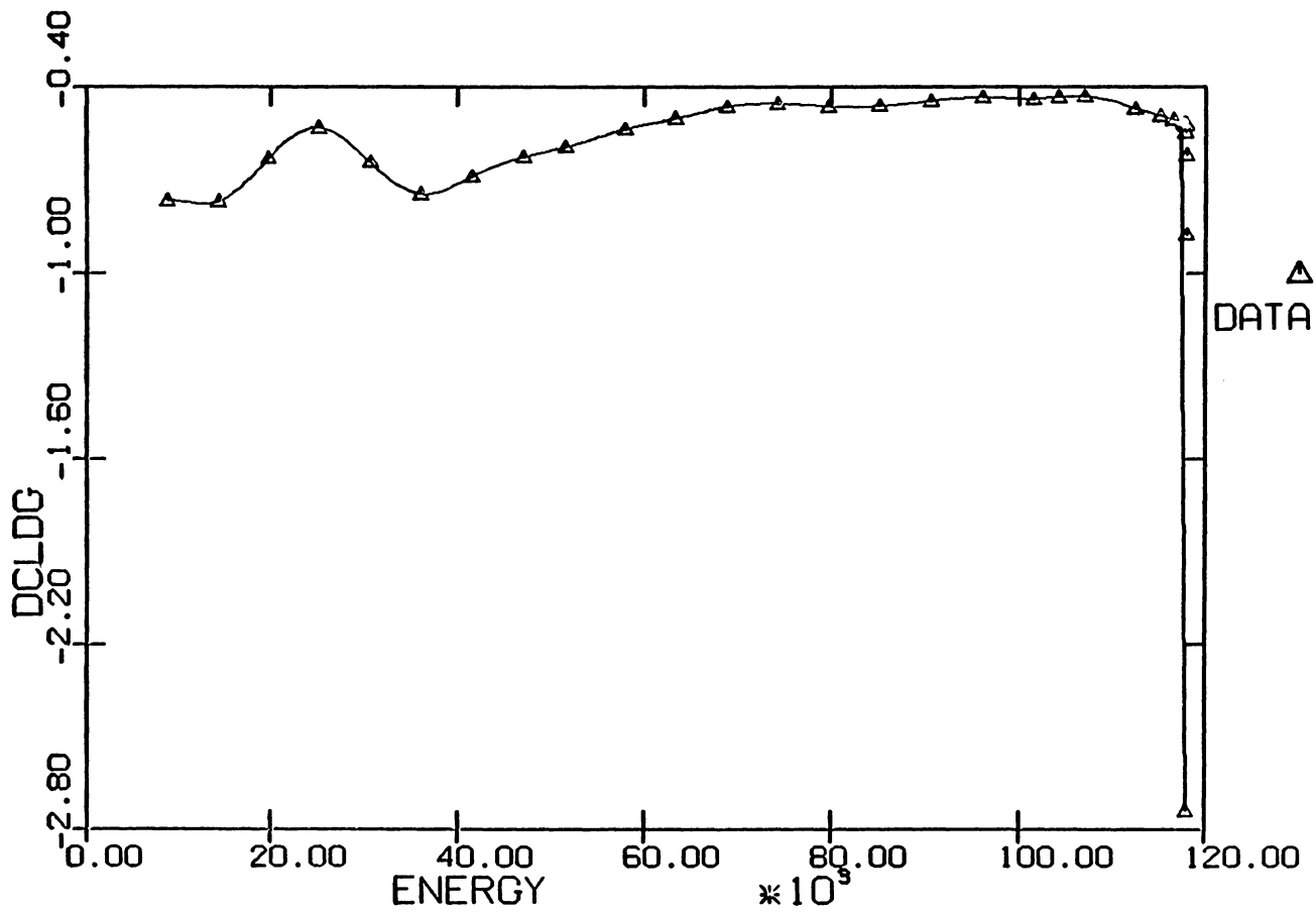
Fig 37.....Path-Angle vs Energy
