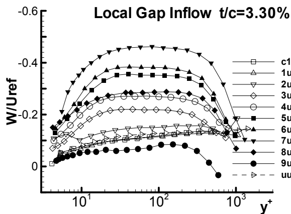
(d) Local Upstream t/c = 3.30\%
