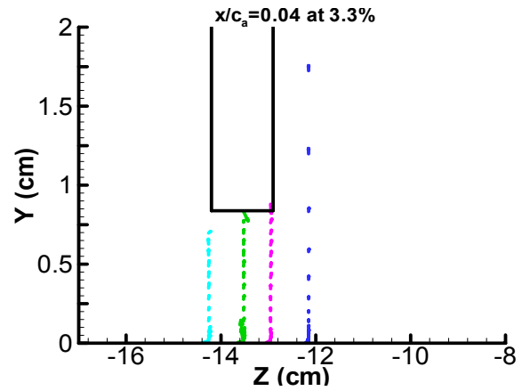
(d) x/c_a = 0.04 t/c = 3.30\%
