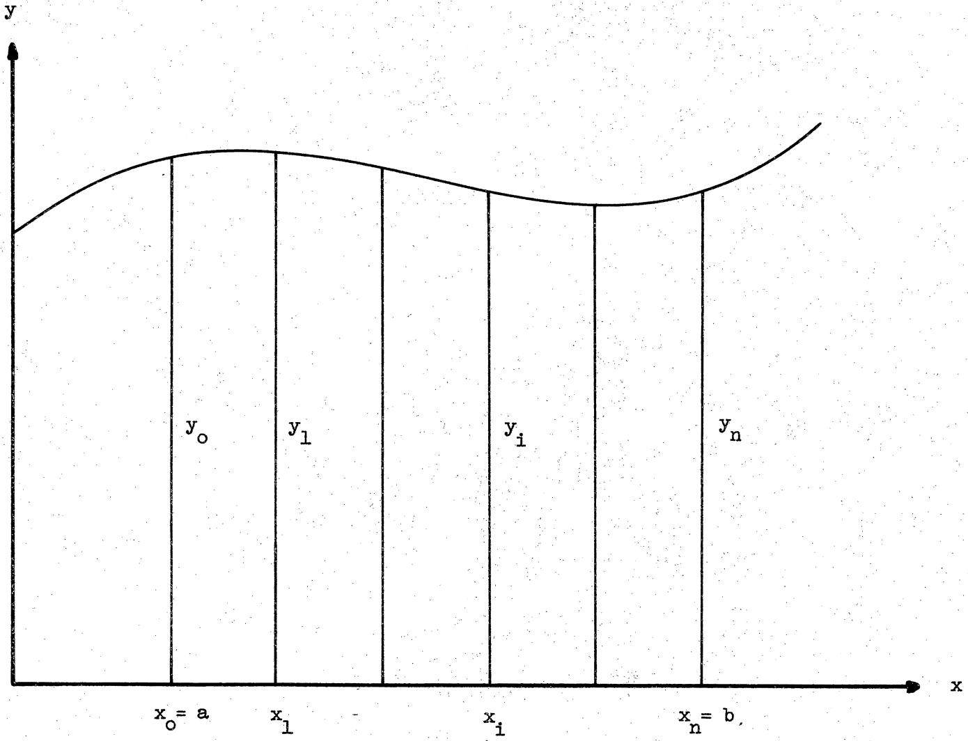
Figure 1.- Function y = f(x) .
