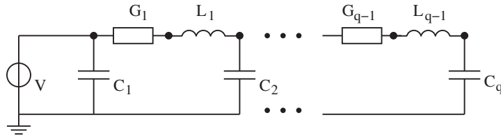
FIG. 2.1. RLC circuit.
