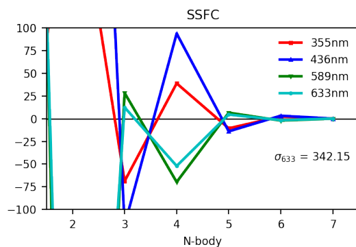
(b) ( S )-methylthiirane
